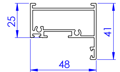
Précadre Battant
