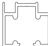
Profil de cadre n°12.216
