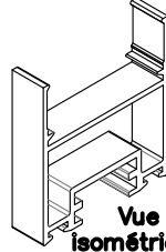
Profil de cadre n°12.216
