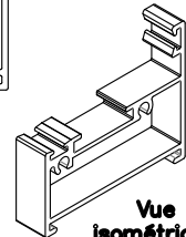
Précadre battant
