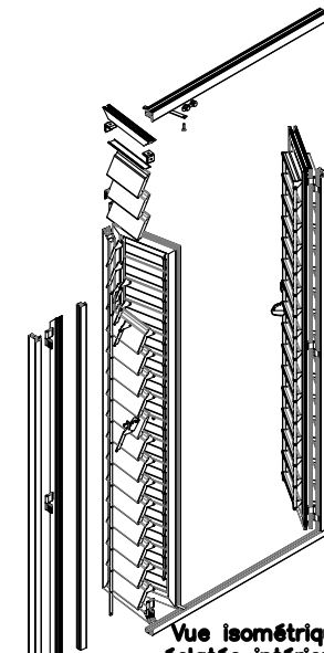
Rail haut pose plafond
