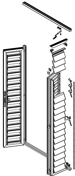
Vue isométrique éclatée extérieure
