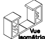
Rail bas pose plafond
