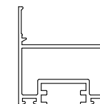
Profil de cadre n°12.216
