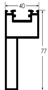
Profil du cadre
