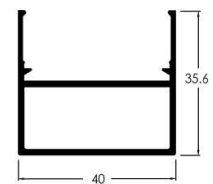
Profil du cadre
