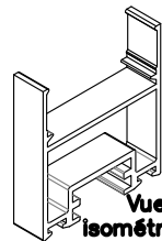
Profil de cadre n°12.216
