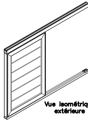
Rail haut 12.996 pose plafond
