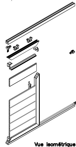
Vue isométrique éclatée extérieure
