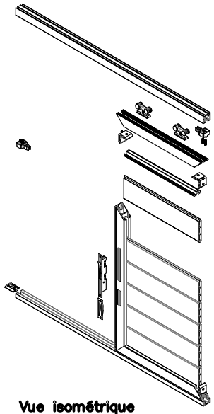
Vue isométrique éclatée intérieure
