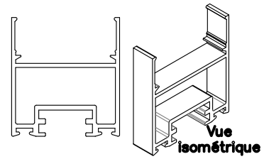
Vue isométrique extérieure Profil de cadre n°12.216
