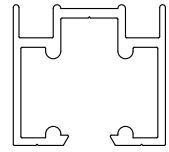
Rail haut pose plafond
