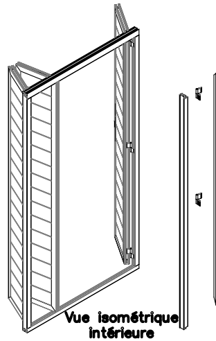
Précadre battant
