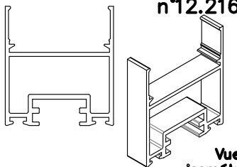
Profil de cadre n°12.216
