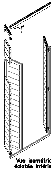
Rail haut pose plafond
