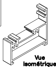
Précadre battant
