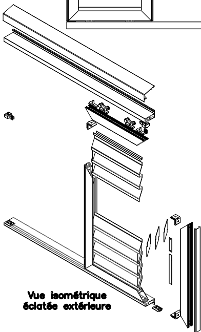
Vue isométrique extérieure
