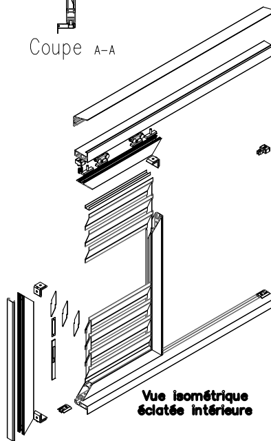
Vue isométrique intérieure
