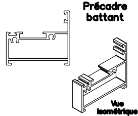
Vue isométrique
