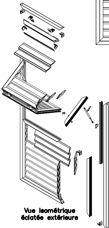
Vue isométrique extérieure
