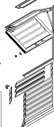
Vue isométrique éclatée intérieure
