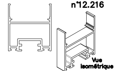
Profil de cadre n°12.216
