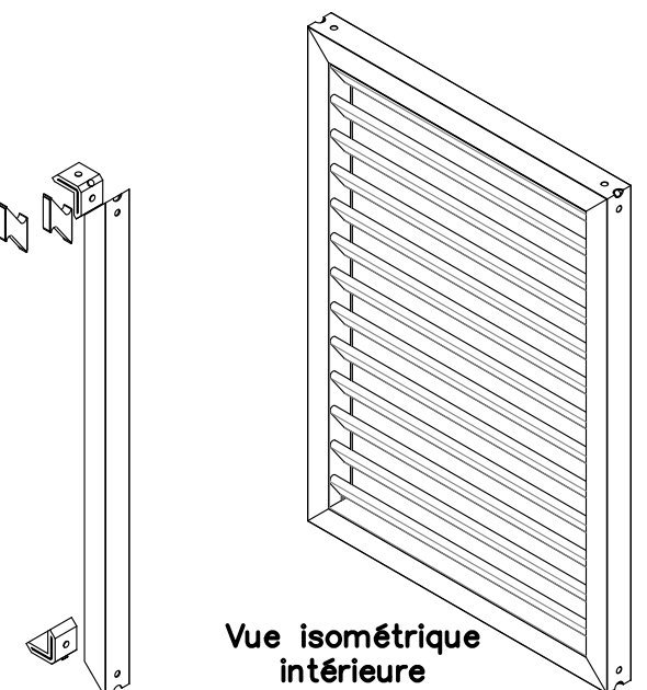
Vue isométrique éclatée intérieure
