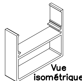
Cadre fixe 35X40
