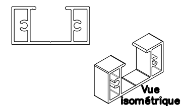
Rail bas 13.117 pose plafond
