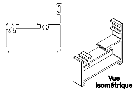
Précadre battant
