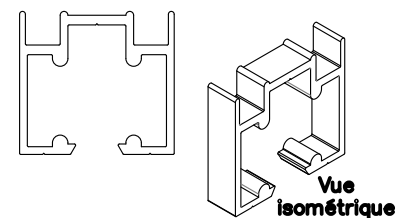
Rail haut 12.996 pose plafond
