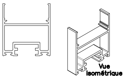
Profil de cadre n°12.216
