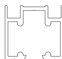
Rail haut 12.996 pose plafond
