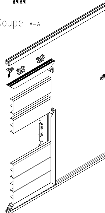
Vue isométrique éclatée extérieure
