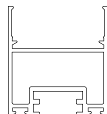
Profil de cadre n°12.216
