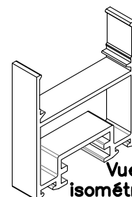
Profil de cadre n°12.216
